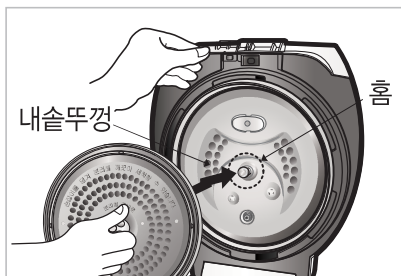
⑥ 뚜껑에 장착시에는 분리형커버 손잡이를 잡고 화살표 방향대로 안쪽의 홈에 맞춘 후 힘주어 눌러주십시오.
